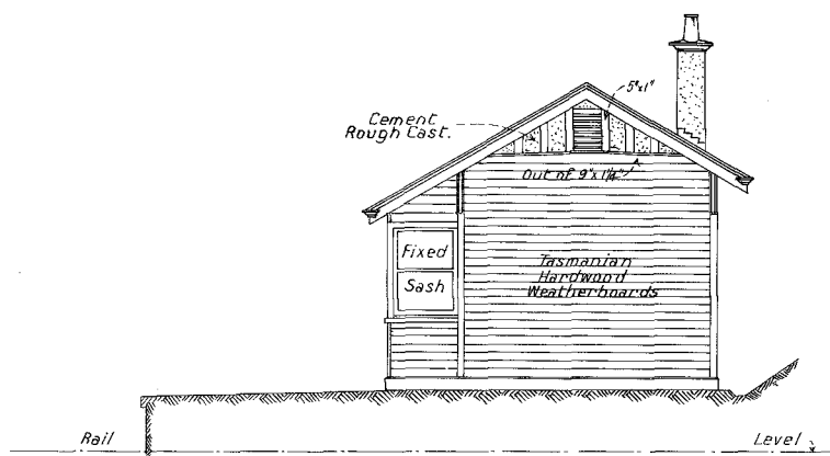
— END ELEVATION —
