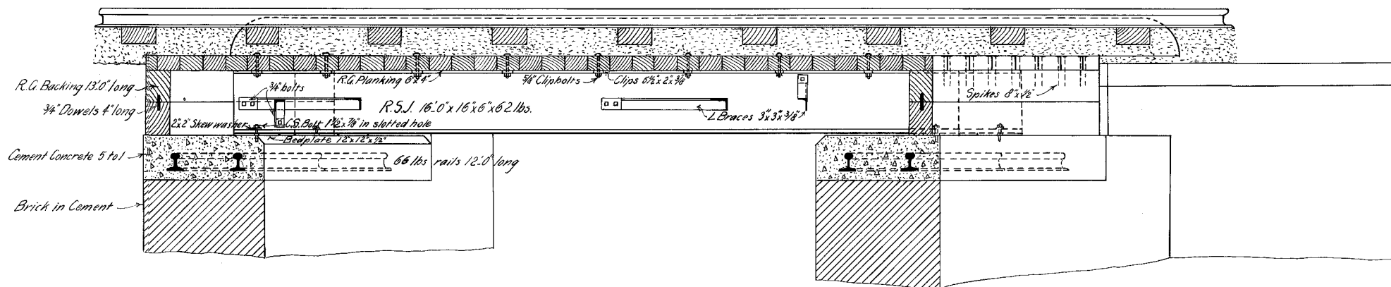
Longitudinal Section
