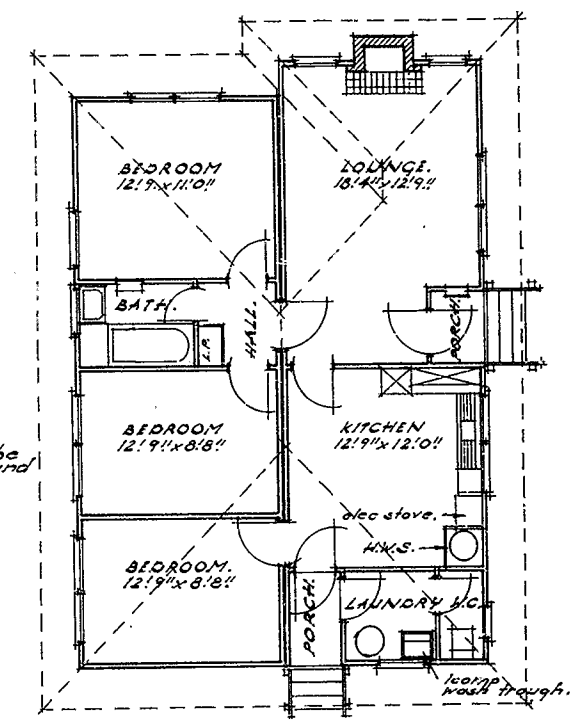
PLAN OF D.R. TYPE A.
