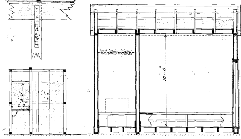
Section C-D
