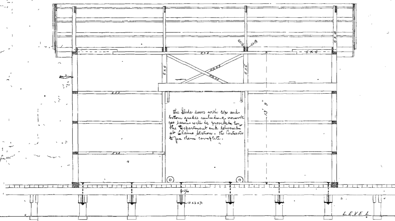
LONGITUDINAL SECTION
