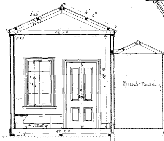
Section A-B
