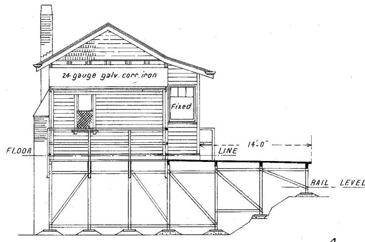
— END ELEVATION —
