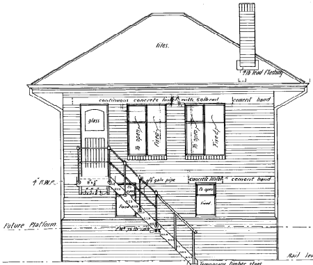
END ELEVATION
